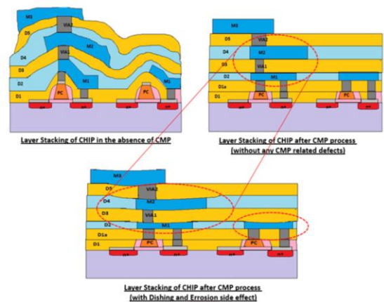
圖 3. CMP 製程為了去除多餘材料或是為電路結構建立完全平坦基底
