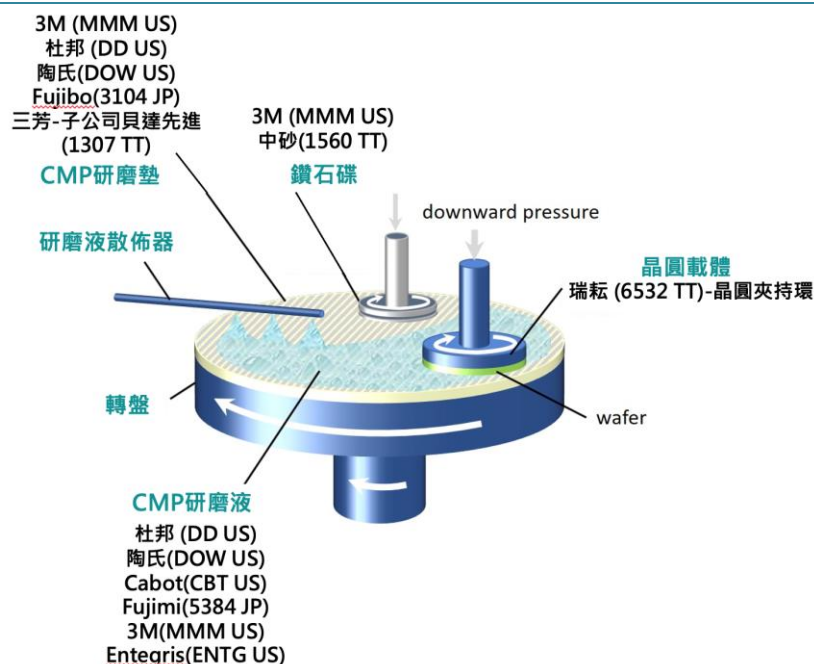
圖 4. CMP 製程各零組件供應商
