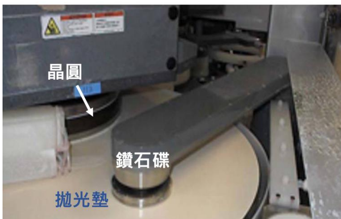
圖 2. CMP 製程實物外觀
